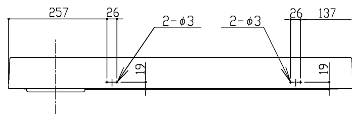
パン本体穴加工位置（現場加工）
