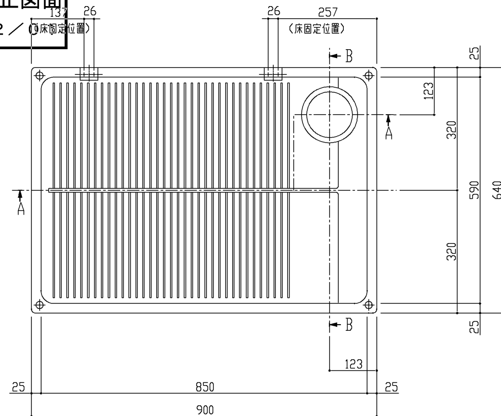
洗濯機設置有効寸法組合せ
